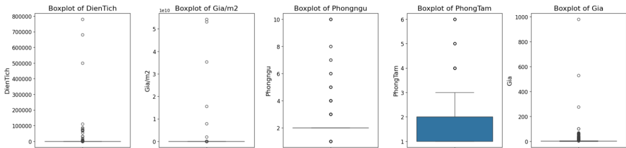
Hình 6. Biểu đồ hộp trước khi xử lý ngoại lệ.
