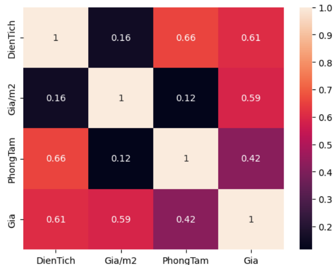
Hình 9. Biểu đồ heatmap thể hiện sự tương quan giữa các biến.
